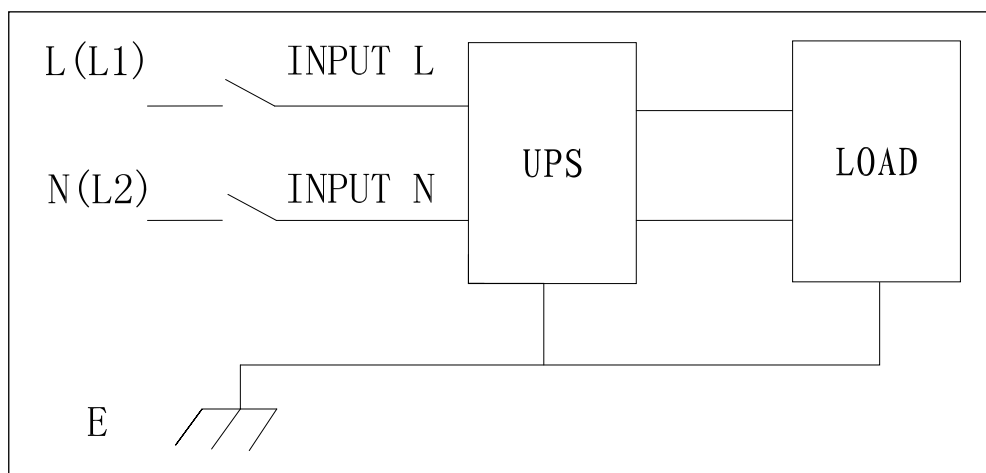
Connessioni Ingresso "monofase + terra"
