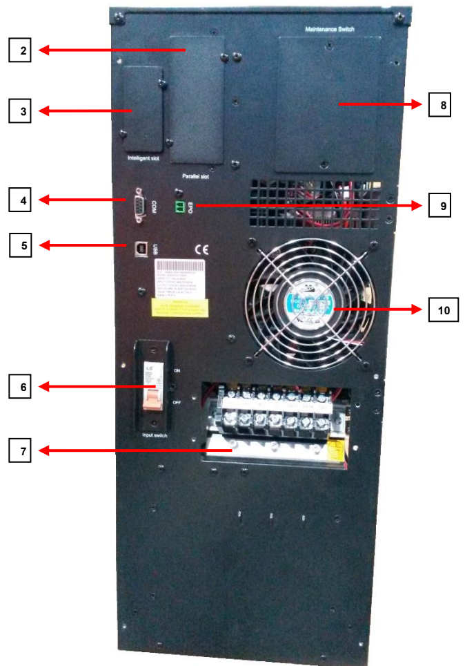
10KVA - Vista posteriore
