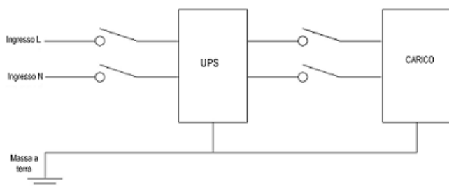
Fig.1 Collegamenti corretti
