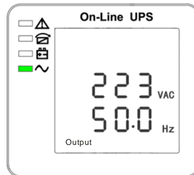
Tensione uscita
