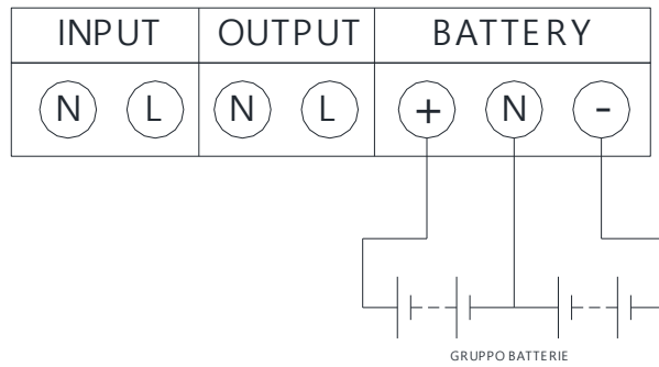
Fig.3 Connessioni morsettiera
