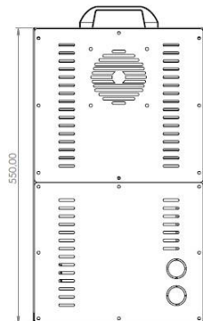
VERSIONE 5KVA
