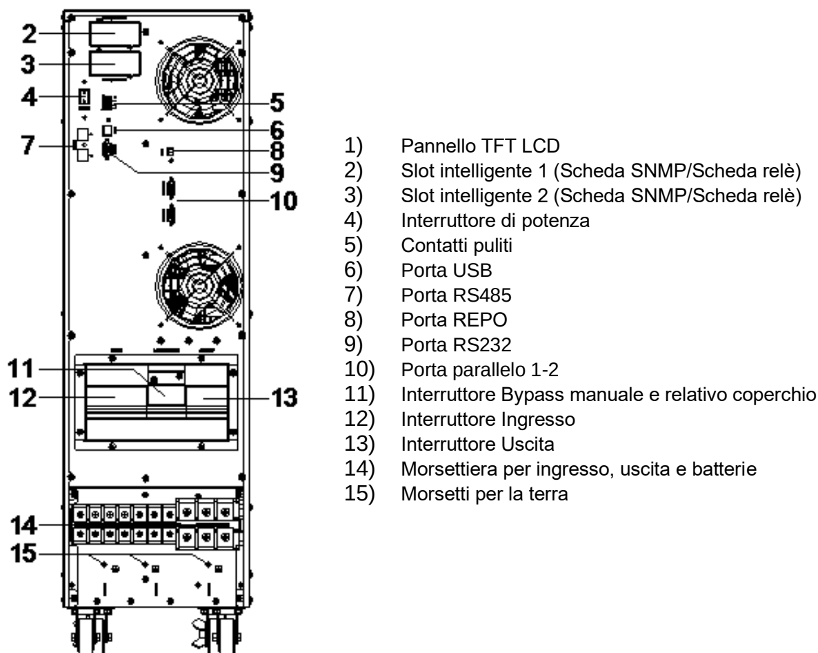
Vista Posteriore 30-40KVA (blocco morsettiera senza coperchio)
