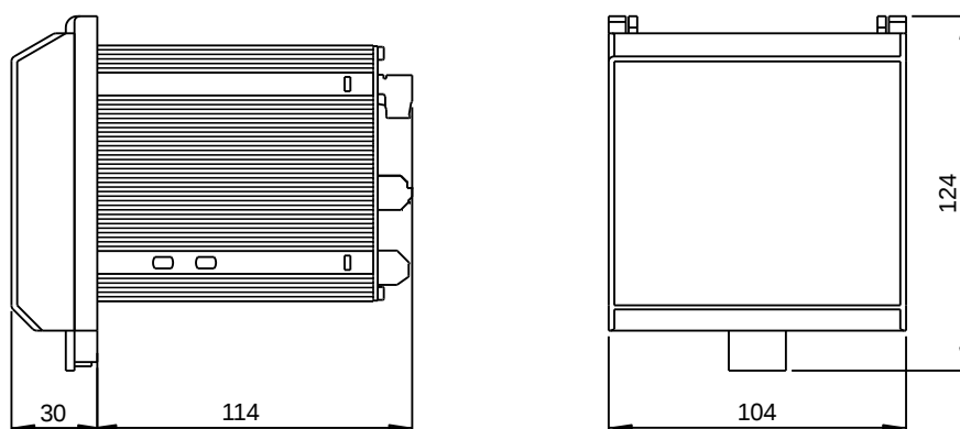
DIMENSIONI VERSIONE IP54
