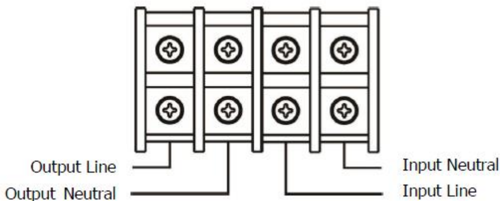
Schema collegamento terminali
