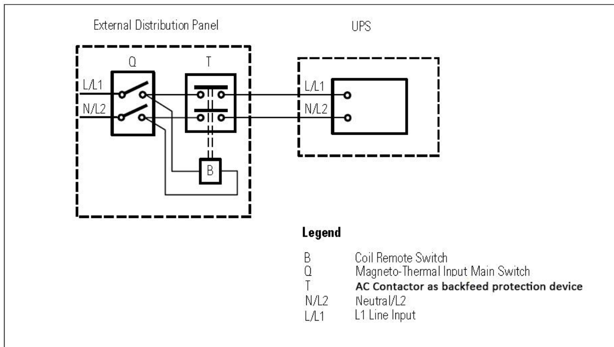
Schema 1: Cablaggio esterno protezione di ritorno
