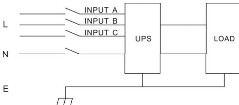
Fig.1 Collegamenti corretti
