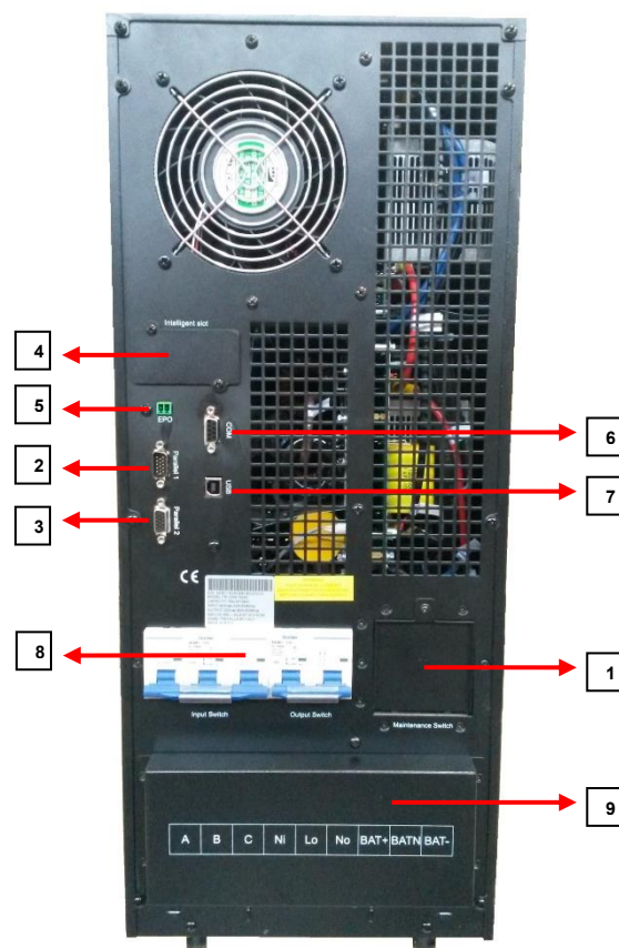
15-20KVA - Vista posteriore
