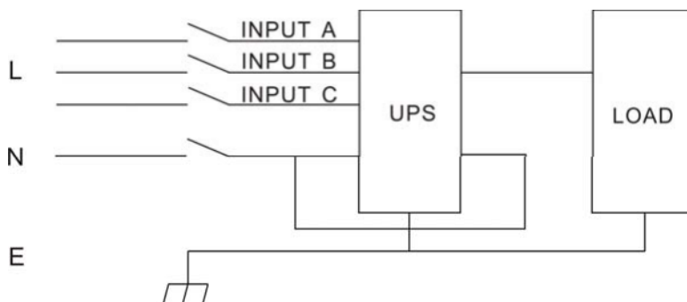
Fig.2 Collegamenti errati
