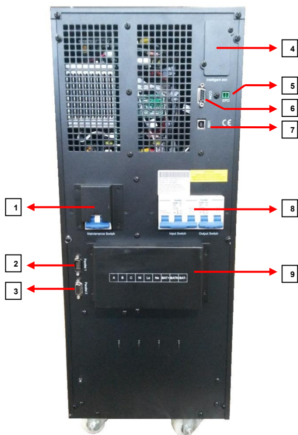
10KVA - Vista posteriore
