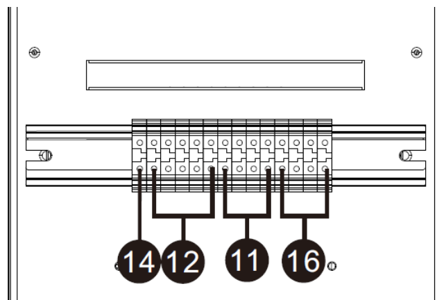
Diagram 2: HV 10K(L)/15K(L)/20K(L)
