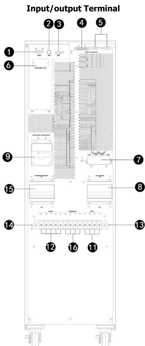
Diagram 3: HV 30K(L)/ LV 15K(L) pannello posteriore
