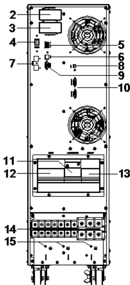
Vista Posteriore 30-200KVA (blocco morsettiera senza coperchio)
