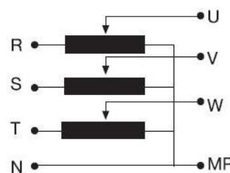
1 - schema di principio
