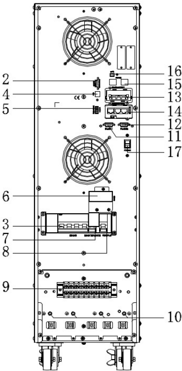
Vista Posteriore 10kVA (morsettiera senza coperchio)
