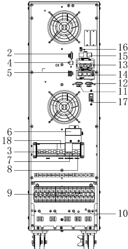
Vista Posteriore 10kVA (Doppio ingresso, morsettiera senza coperchio)
