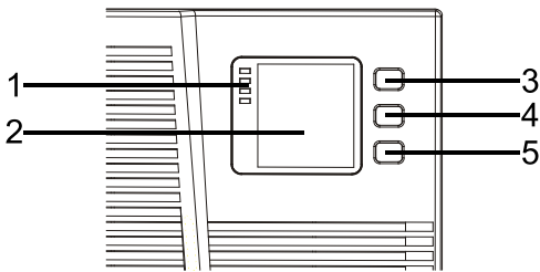
Pannello di controllo LCD introduzione
